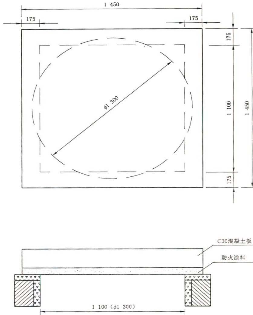
图3 耐火试件安装
